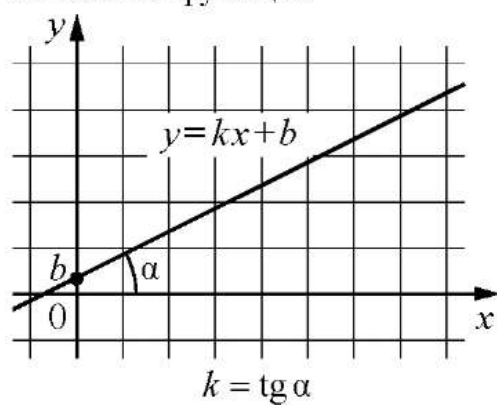
Линейная функция
