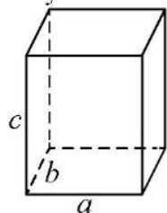
Прямоугольный параллелепипед
