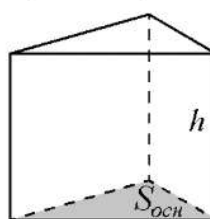
Прямая призма
