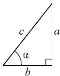
Прямоугольный треугольник
