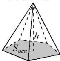
Пирамида
