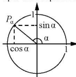
Тригонометрическая окружность
