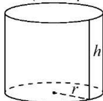
Цилиндр
